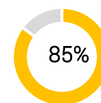
Plaquages Réussis %
