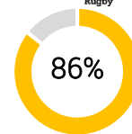
Efficacité Percussion %
